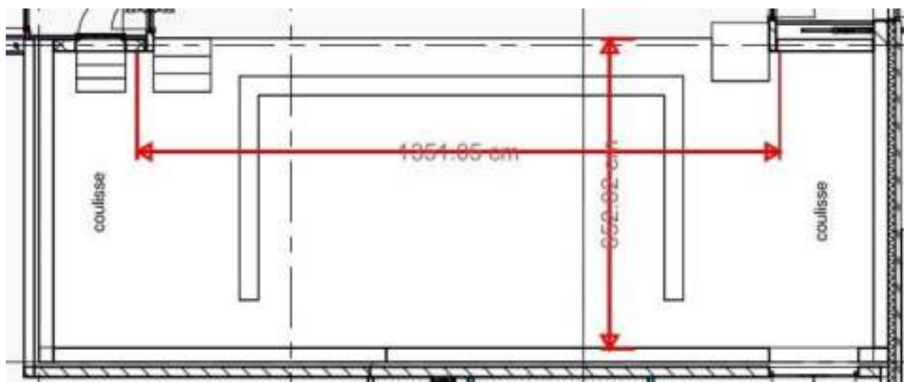
Podium bovenaanzicht
